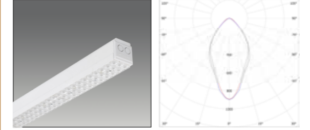
60° Optik Lensli Aydınlatma Armatürü
