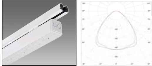
90° Optik Lensli Aydınlatma Armatürü
