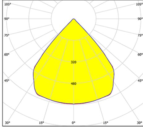
80° - White Reflector
