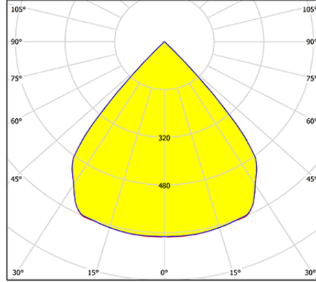
80° - Black Reflector
