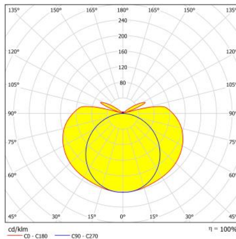
SP 1500 AYN
